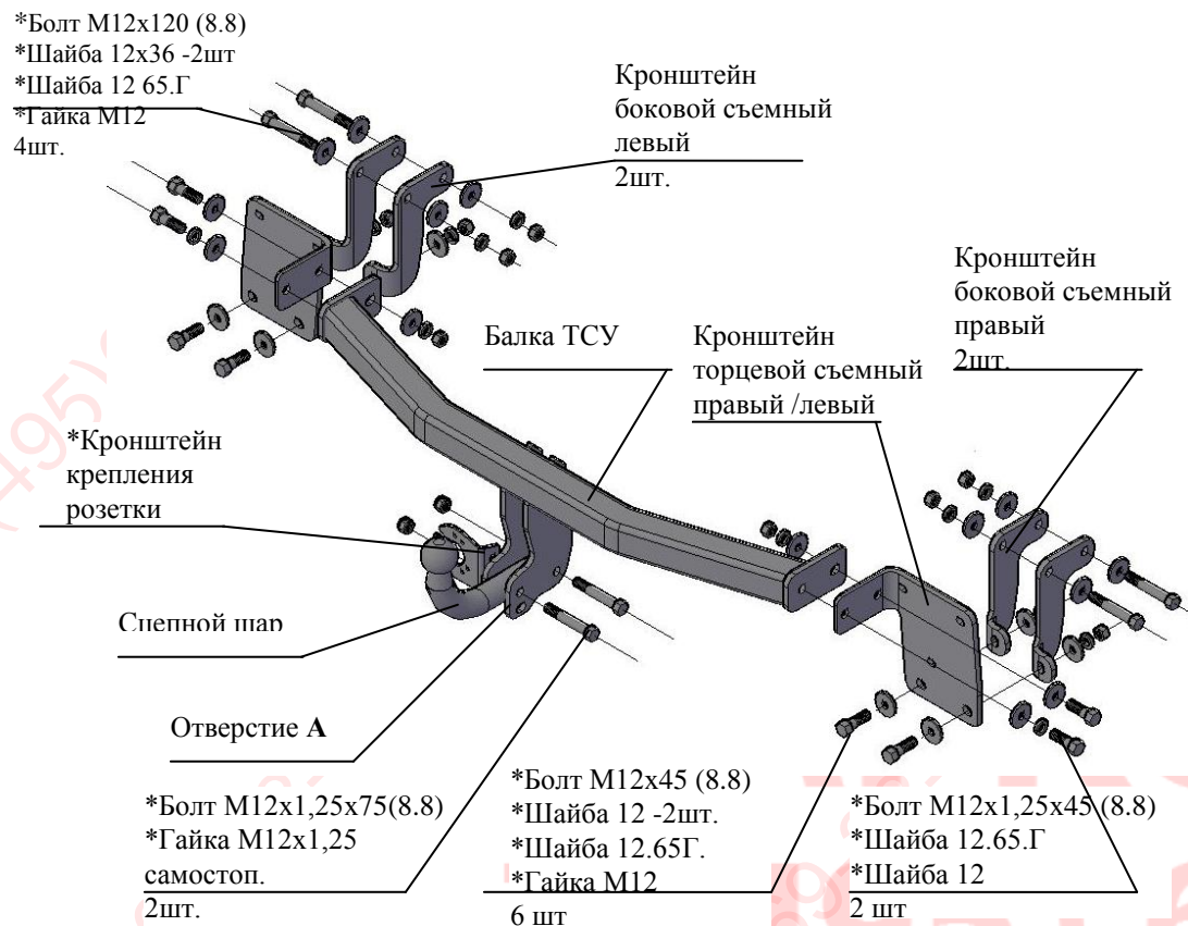
Рис.1 Тягово-сцепное устройство 7140
