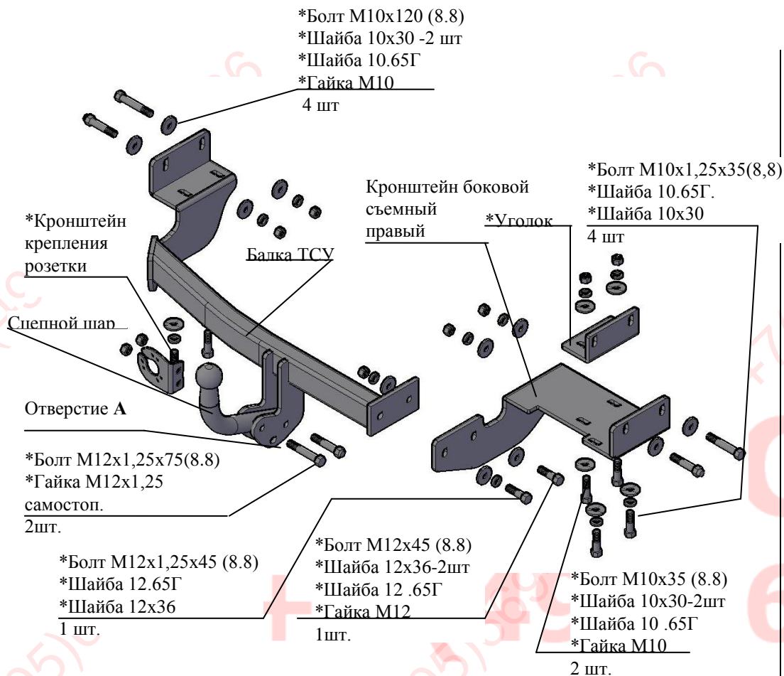
Рис.1 Тягово-сцепное устройство 7360
