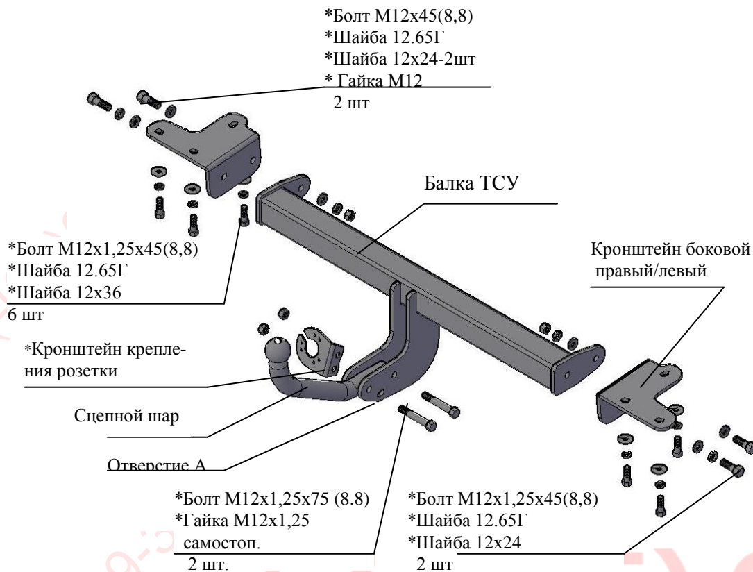
Рис.1 Тягово-сцепное устройство 7900.
