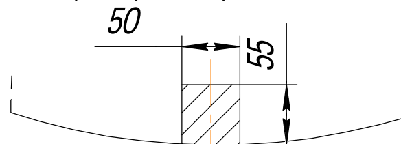
Подрезка края бампера для Santa Fe 2018-
