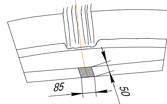
Эскиз подрезки бампера
