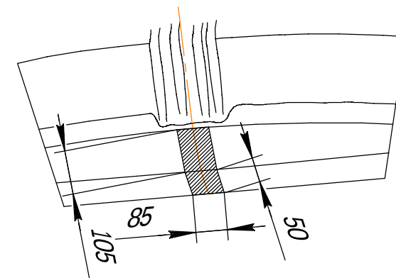
Эскиз подрезки бампера
