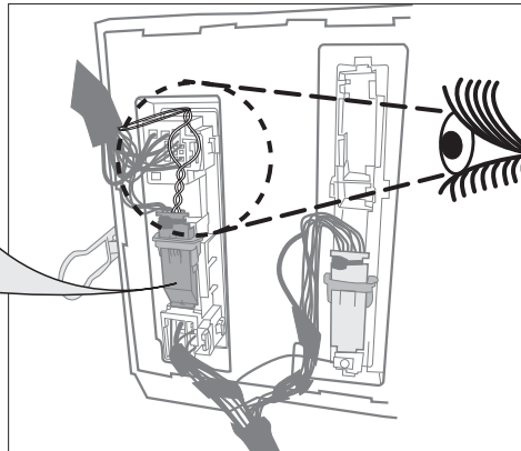
Steckhülsegehäuse 32-polig (BK) Connector 32-pin (BK)
