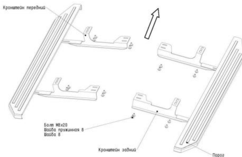
Рис. 1 Схема установки комплекта порогов
