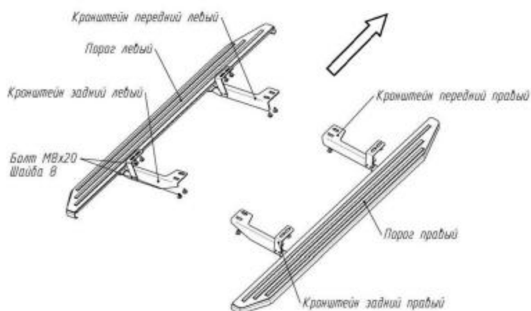
Рис. 1 Схема установки комплекта порогов
