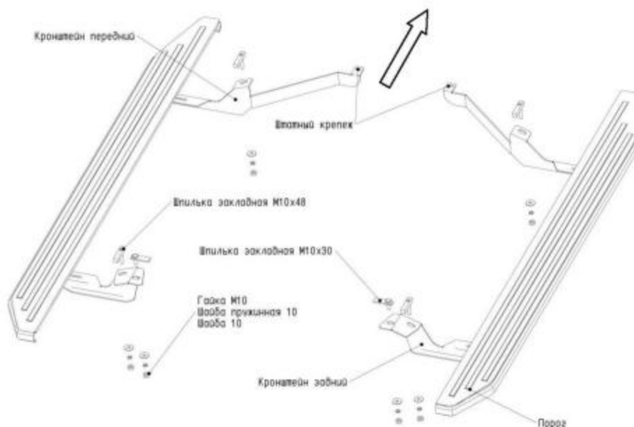
Рис. 1 Схема установки комплекта порогов
