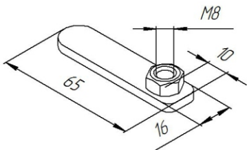
Закладной кронштейн с гайкой
