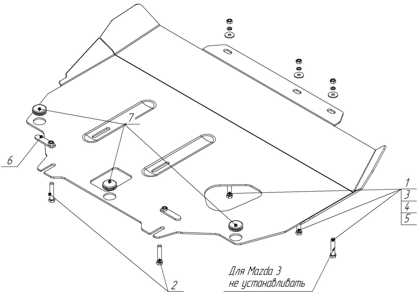
Закладной кронштейн с гайкой
