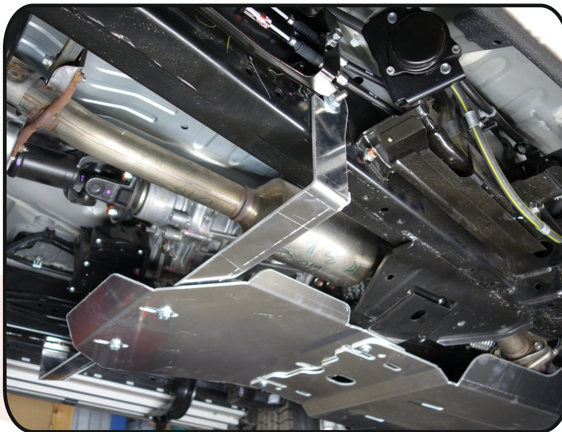
Защита раздатки (алюминий) 4 мм арт. ZKTCC00049
