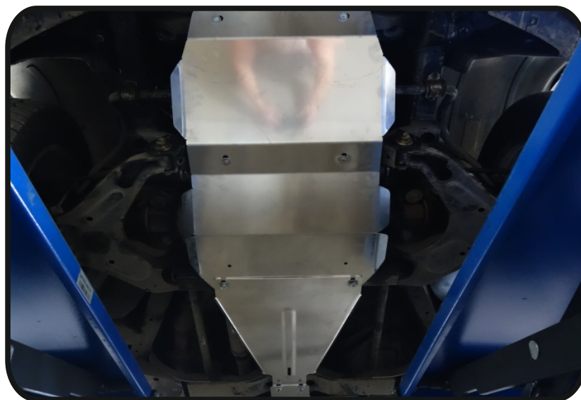
Защита картера (алюминий) 4мм арт.ZKTCC00087
