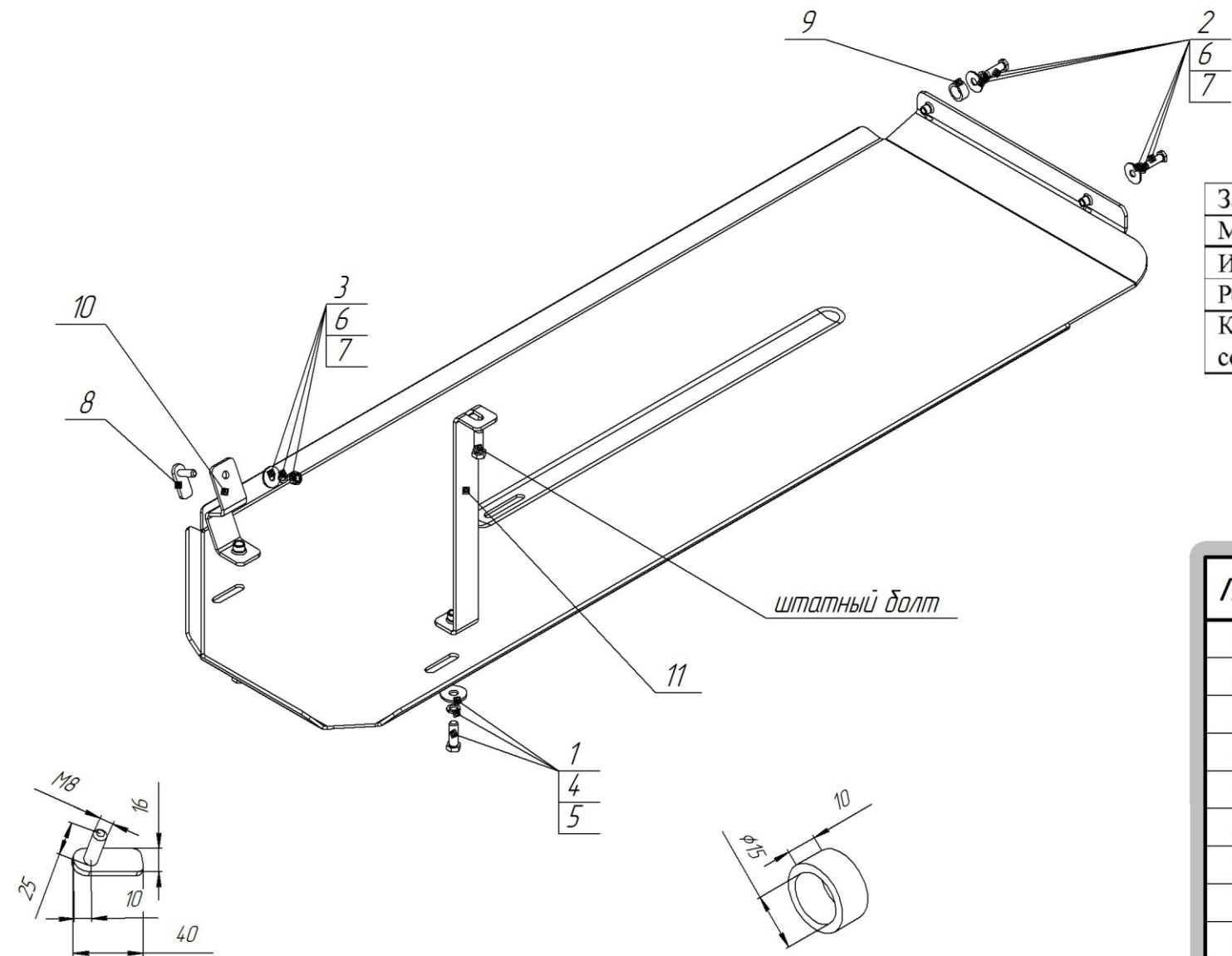
Кронштейн закладной М8х25 (поз.8)
