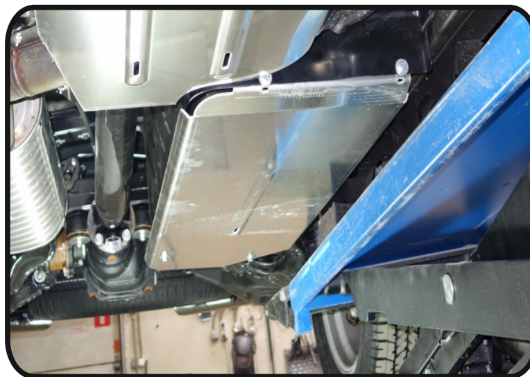
Защита бака (алюминий) 4мм арт.ZKTCC00110
