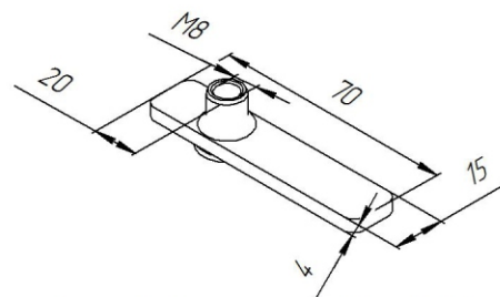
Закладной кронштейн M8 70x15
