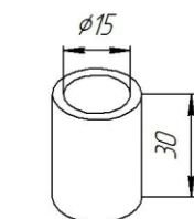
Втулка L=30 мм
