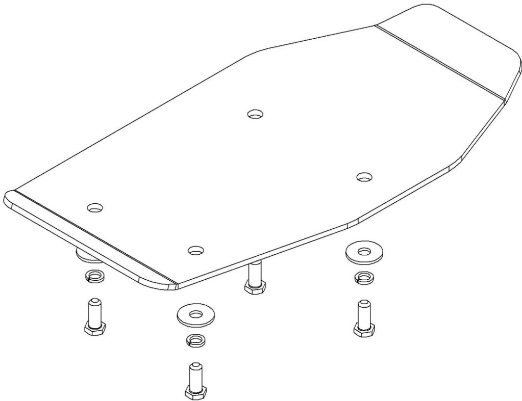
Схема установки
