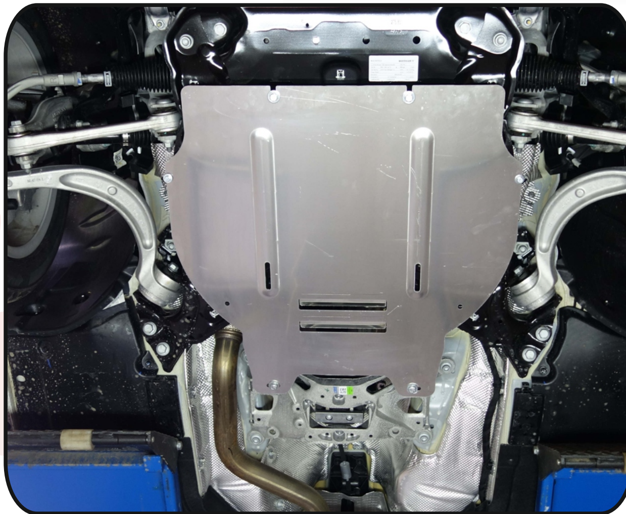
Защита КПП (алюминий) 4 мм арт. ZKTCC00190
