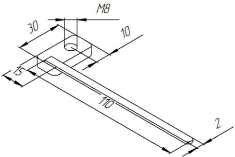
Закладной кронштейн (поз.7)
