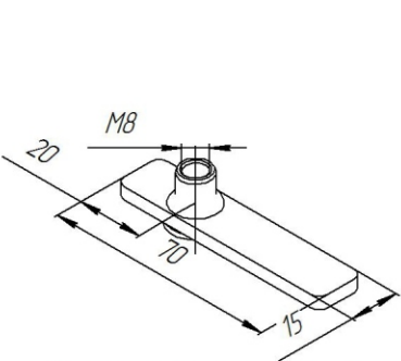
Кронштейн закладной с заклепкой М8 (поз.6)
