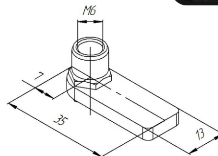
Кронштейн поз. 4
