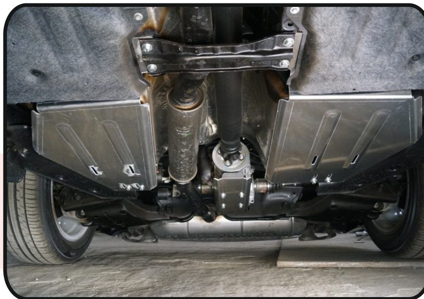
Защита бака (алюминий) 4 мм (комплект 2 шт) арт. ZKTCC00367.
