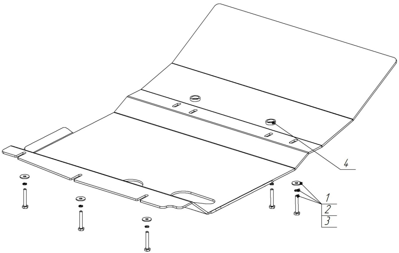
Схема установки
