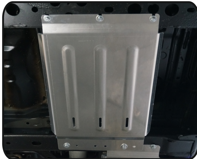
Защита раздаточной коробки (алюминий) 4мм арт.ZKTCC00372.
