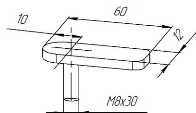
Кронштейн z-32 M8x30_10
