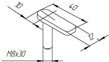
Закладной кронштейн М8 (z-8 М8х30_10)
