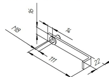
Закладной кронштейн (z-75 M8_14)
