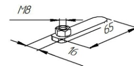
Закладной кронштейн Z47
