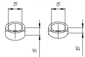
Закладной кронштейн Z47
