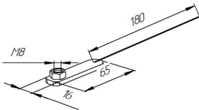
Закладной кронштейн Z47 Φ180мм
