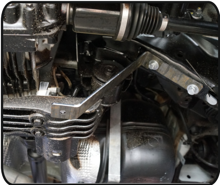
Закладной кронштейн Z47 Φ180мм
