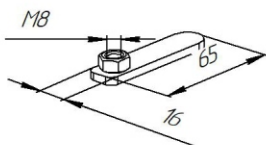
Закладной кронштейн Z47
