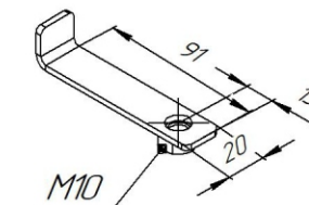
Закладной кронштейн (z-64 M10)
