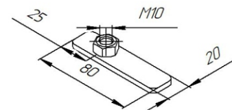
Закладной кронштейн (z-60 M10_25)
