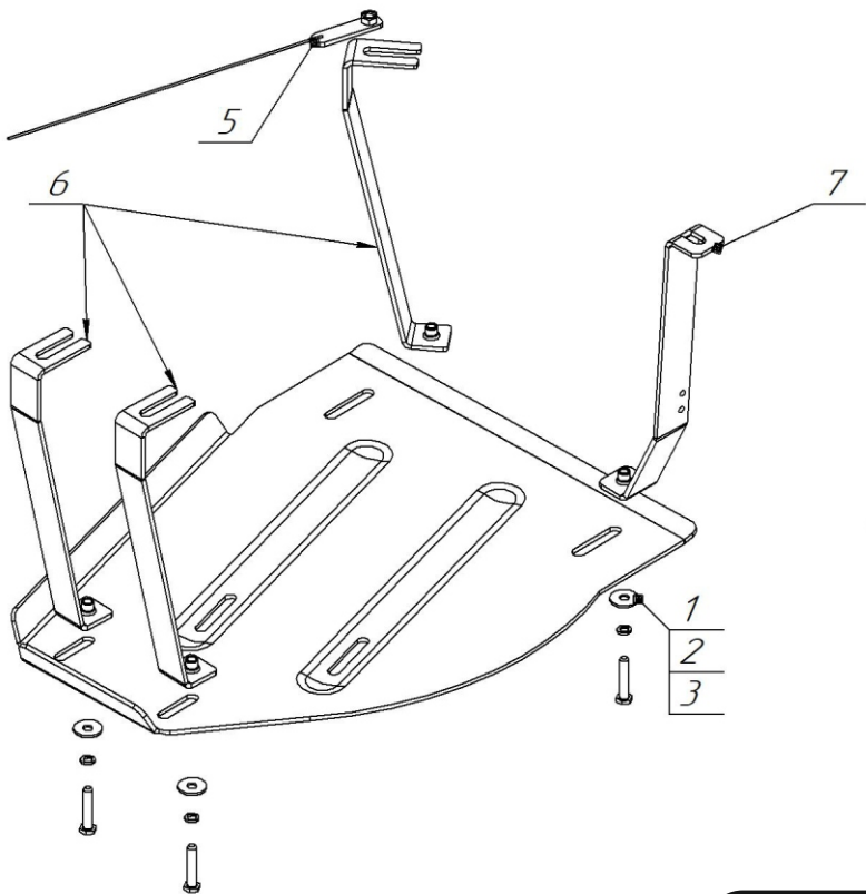
Закладной кронштейн z-47 M8_10_ф2х300 СБ
