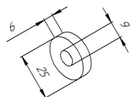
Кронштейн 1665
