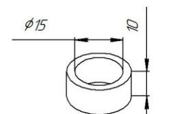
Втулка L=10 мм
