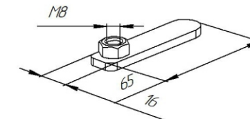
Закладной кронштейн Z47
