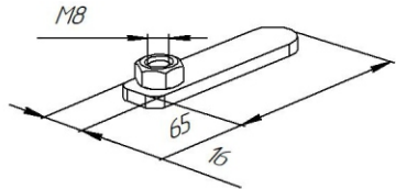
Закладной кронштейн Z47
