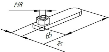
Закладной кронштейн Z47
