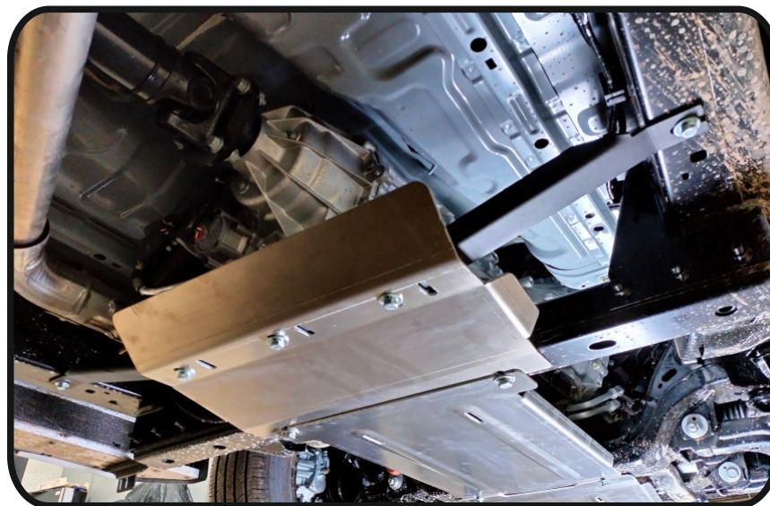
Защита раздаточной коробки (алюминий) 4мм арт.ZKTCC00642.
