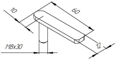
Закладной кронштейн М8х30 (поз.5)
