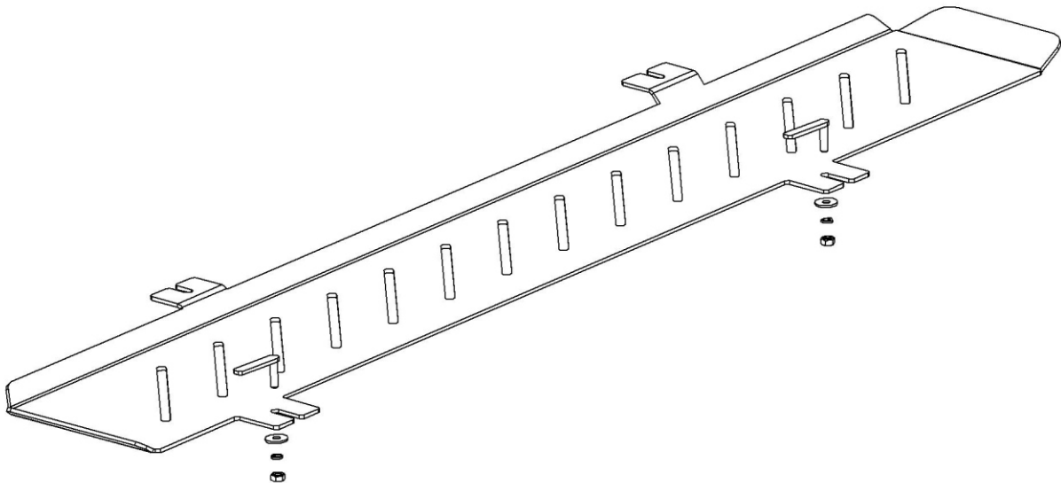
Закладной кронштейн М8х30 (поз.5)
