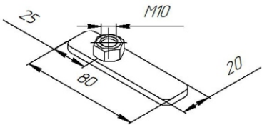
Закладной кронштейн (z-60 M10_25)
