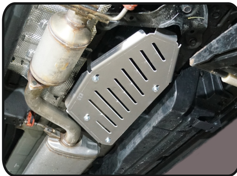
Защита топливопровода (алюминий) 4 мм арт.ZKTCC00668.
