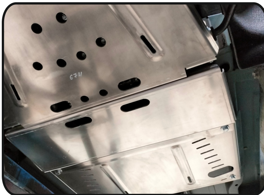
Защита КПП (алюминий) 4мм арт.ZKTCC00675.
