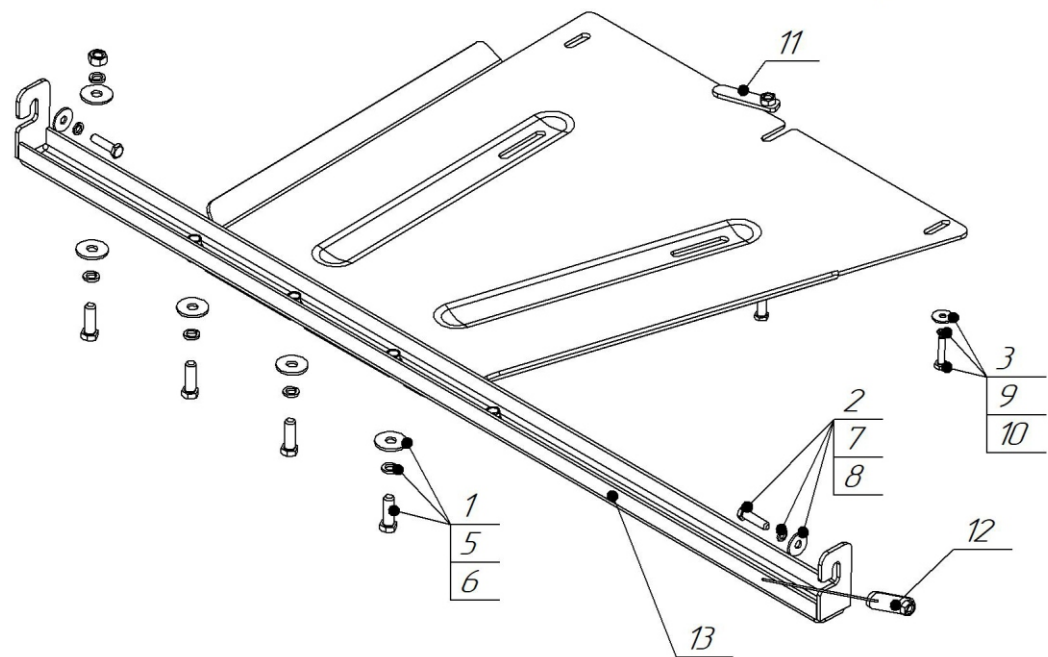
Схема установки
