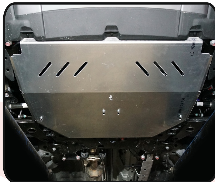
Защита картера и АКПП (алюминий) 4 мм арт. ZKTCC00694.
