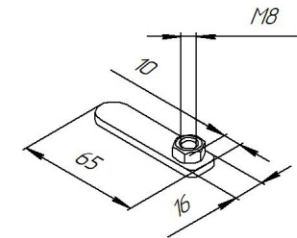
Закладной кронштейн Z47
