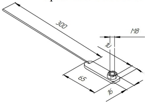
Закладной кронштейн z-47 M8_10_φ2x300 CB
