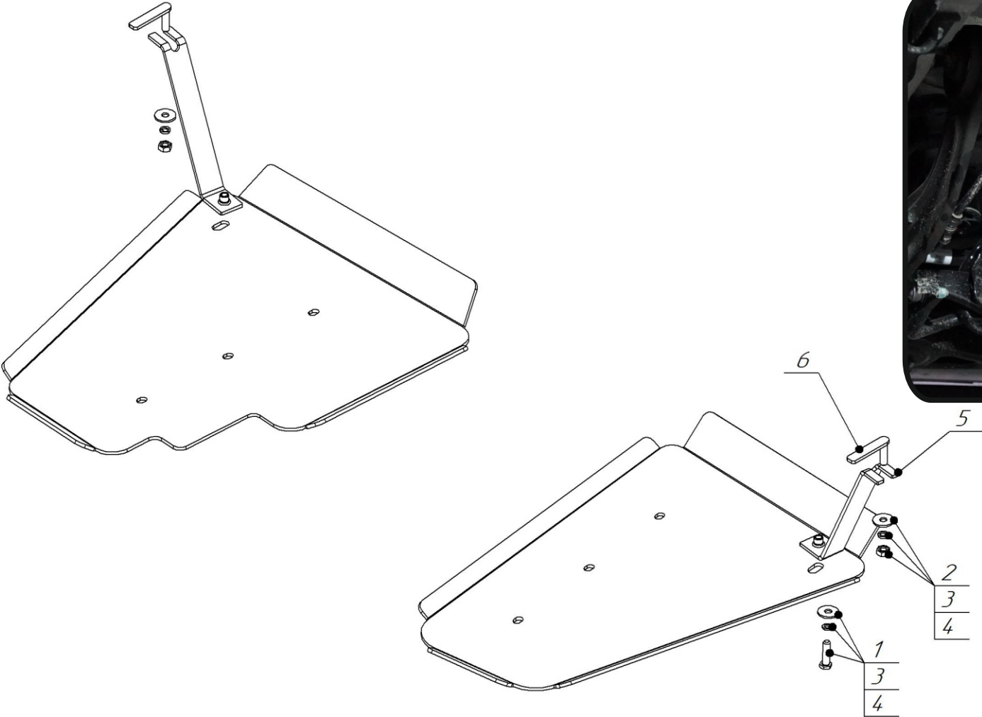
Схема установки
